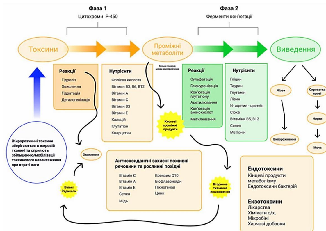
Рис.1. Фази біотрансформації ксенобіотиків
