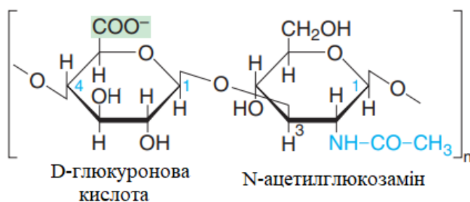
Рис. 1. Структурна формула гіалуронової кислоти.
