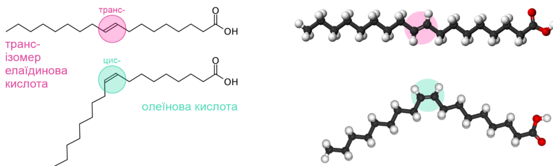
Рис. 2 Приклад транс- і цис- ізомерів омега-9 ненасичених жирних кислот: олеїнова кислота та її транс-ізомер елаїдинова кислота
